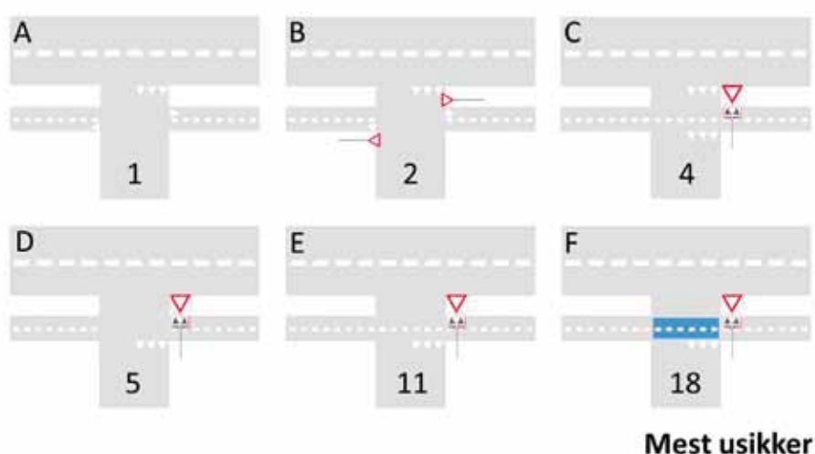
Figur 2. Resultat af uheldsmodel. Uheldsrisikoen for B-F sat i forhold til A.
